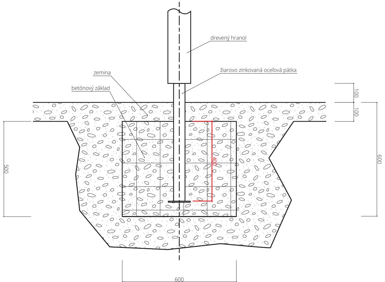
Detail ukotvenia
